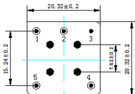
底视图
